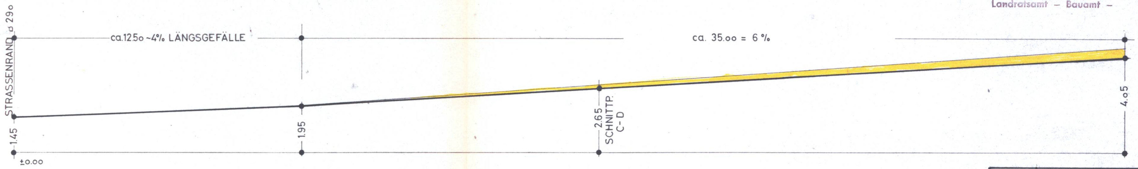
STRASSENLÄNGSSCHNITT A-B
