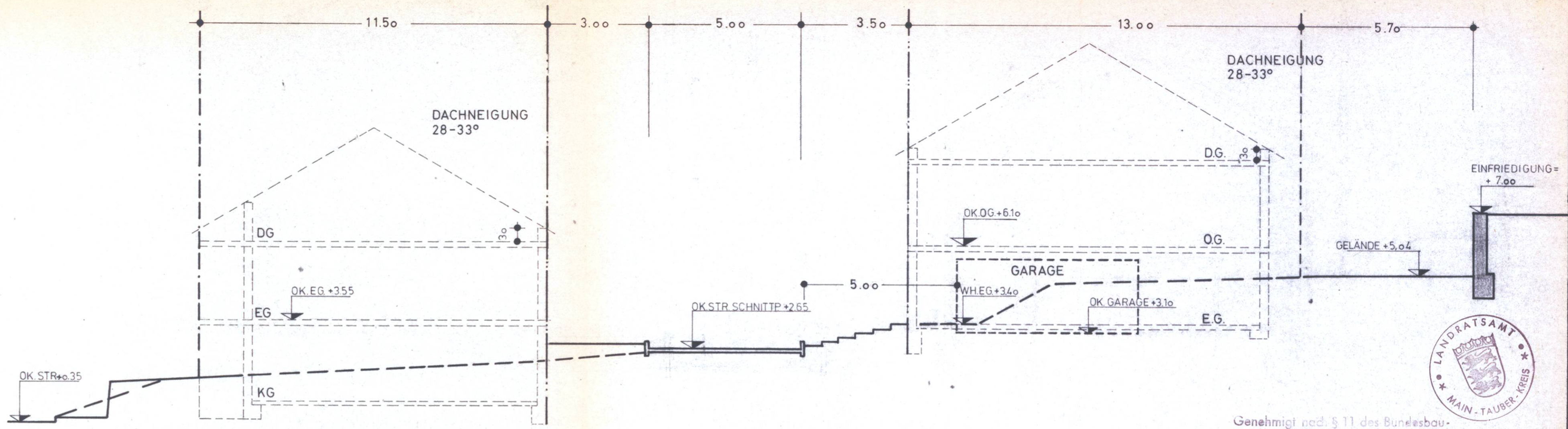
QUERSCHNITT C-D
